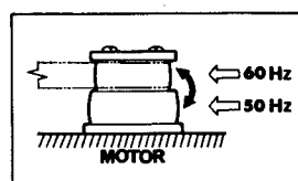
Fig. 10-5 Motor Pulley
